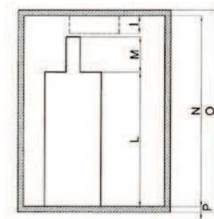
VUE LATÉRALE
